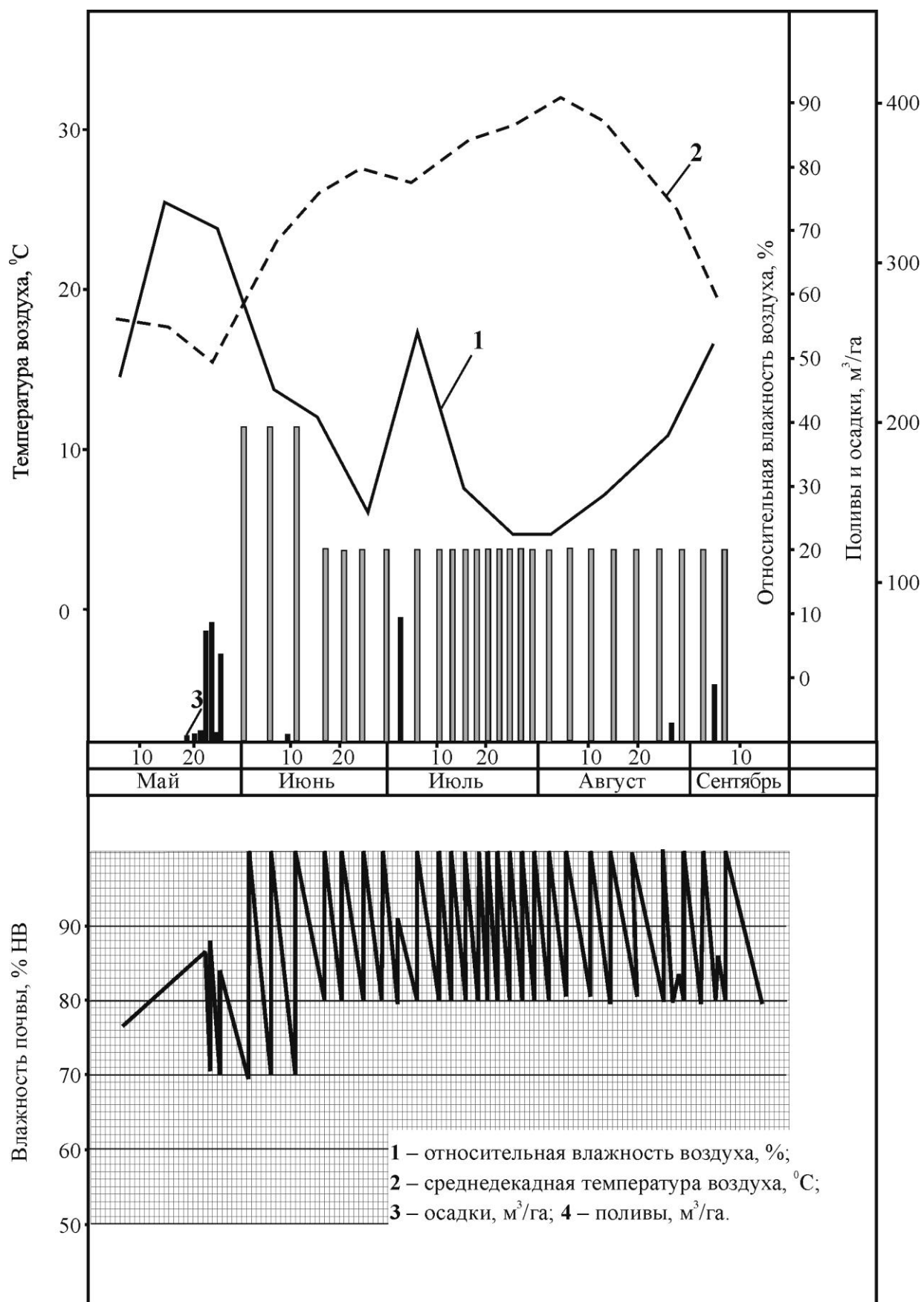
Рисунок 5.7 - Динамика изменения влагосодержания увлажняемой зоны почвогрунта в посевах сои ВНИИОЗ 31 для варианта поддержания предполивной влажности почвы 70-80-80 НВ (2010 г.)
