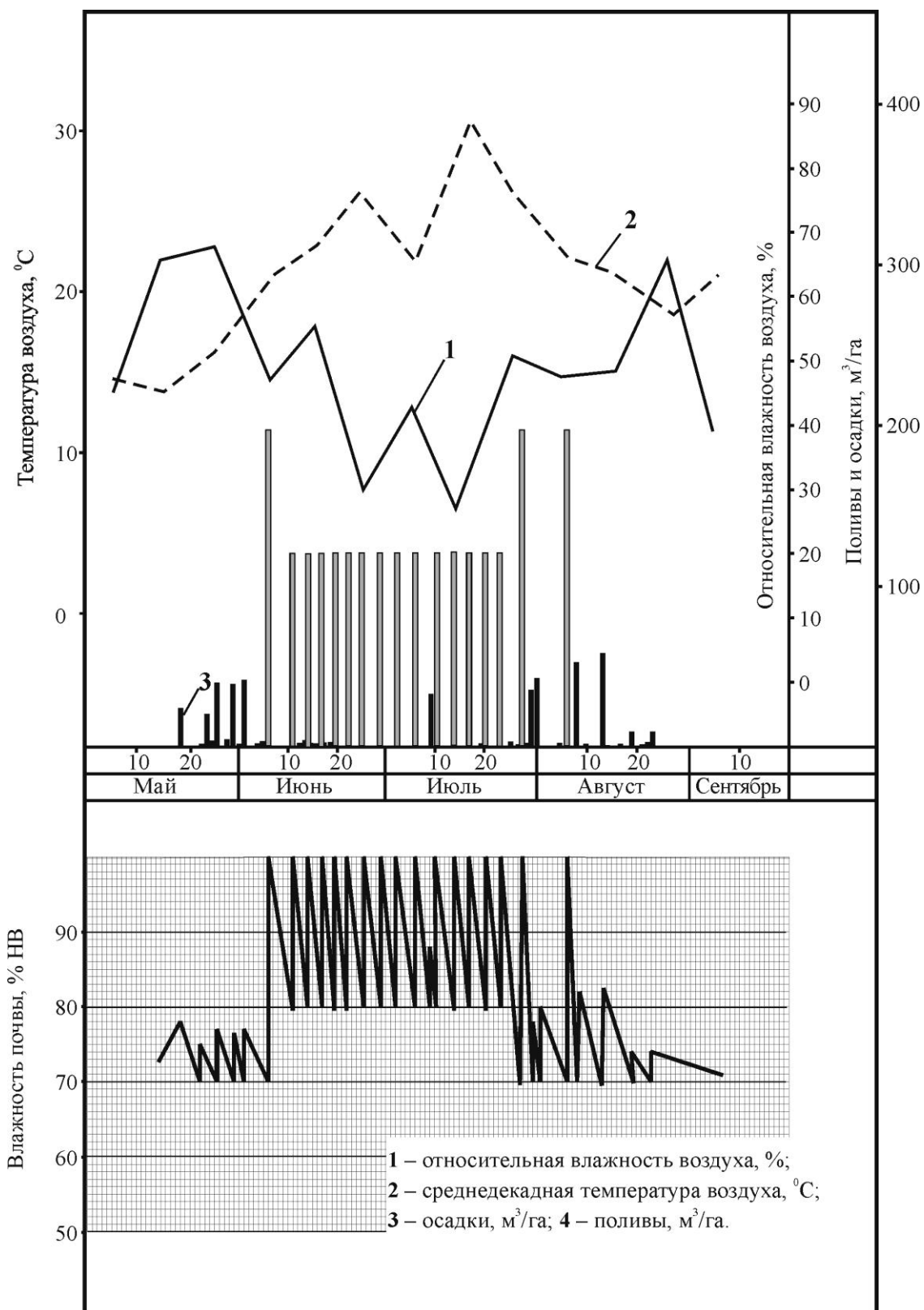
Рисунок 5. 4 - Динамика изменения влагосодержания увлажняемой зоны почвогрунта в посевах сои ВНИИОЗ 86 для варианта поддержания предполивной влажности почвы 70-80-70 НВ (2009 г.)
