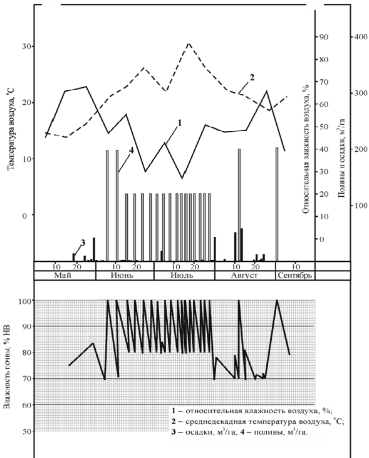
Рисунок 5.1 Динамика изменения влагосодержания увлажняемой зоны почвогрунта в посевах сои ВНИИОЗ 31 для варианта поддержания предполивной влажности почвы 70-80-70 НВ (2009 г.)
