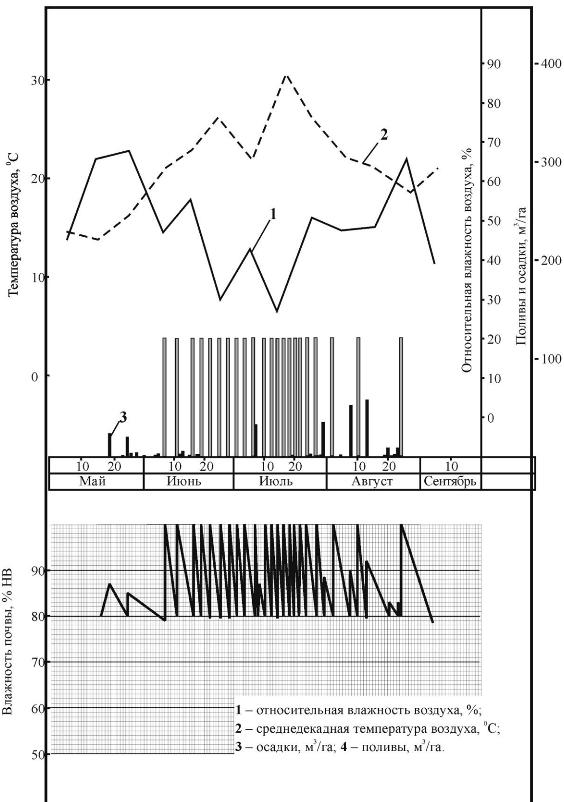
Рисунок 5.3 - Динамика изменения влагосодержания увлажняемой зоны почвогрунта в посевах сои ВНИИОЗ 31 для варианта поддержания предполивной влажности почвы 80-80-80 НВ (2009 г.)
