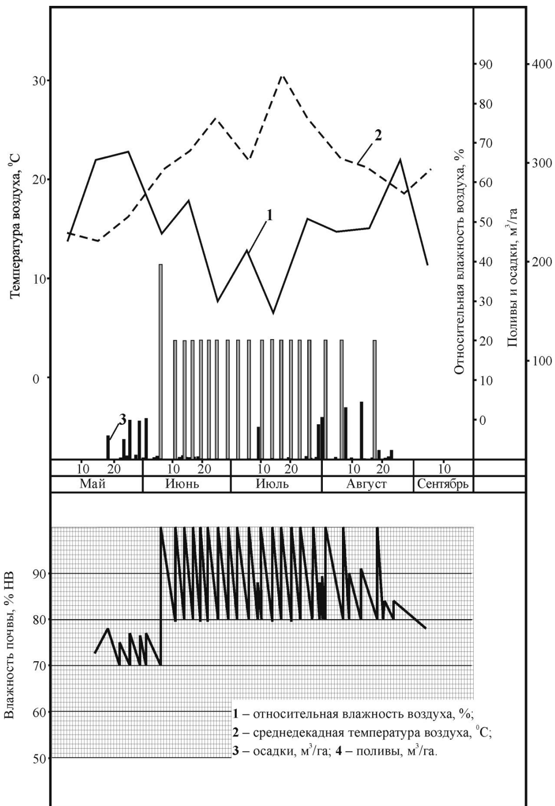
Рисунок 5.2 - Динамика изменения влагосодержания увлажняемой зоны почвогрунта в посевах сои ВНИИОЗ 31 для варианта поддержания предполивной влажности почвы 70-80-80 НВ (2009 г.)
