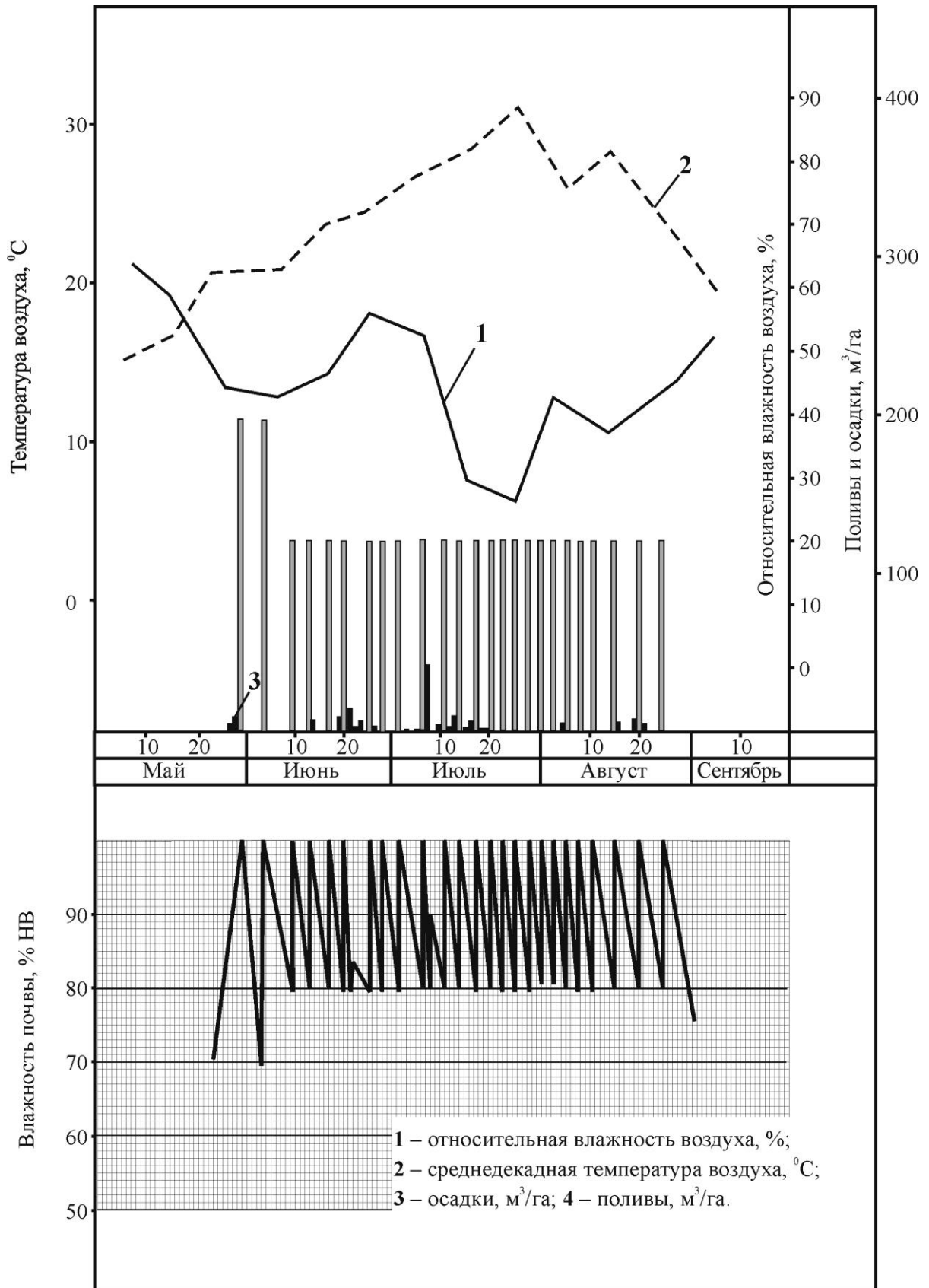
Рисунок 5.10 - Динамика изменения влагосодержания увлажняемой зоны почвогрунта в посевах сои ВНИИОЗ 86 для варианта поддержания предполивной влажности почвы 70-80-80 НВ (2011 г.)
