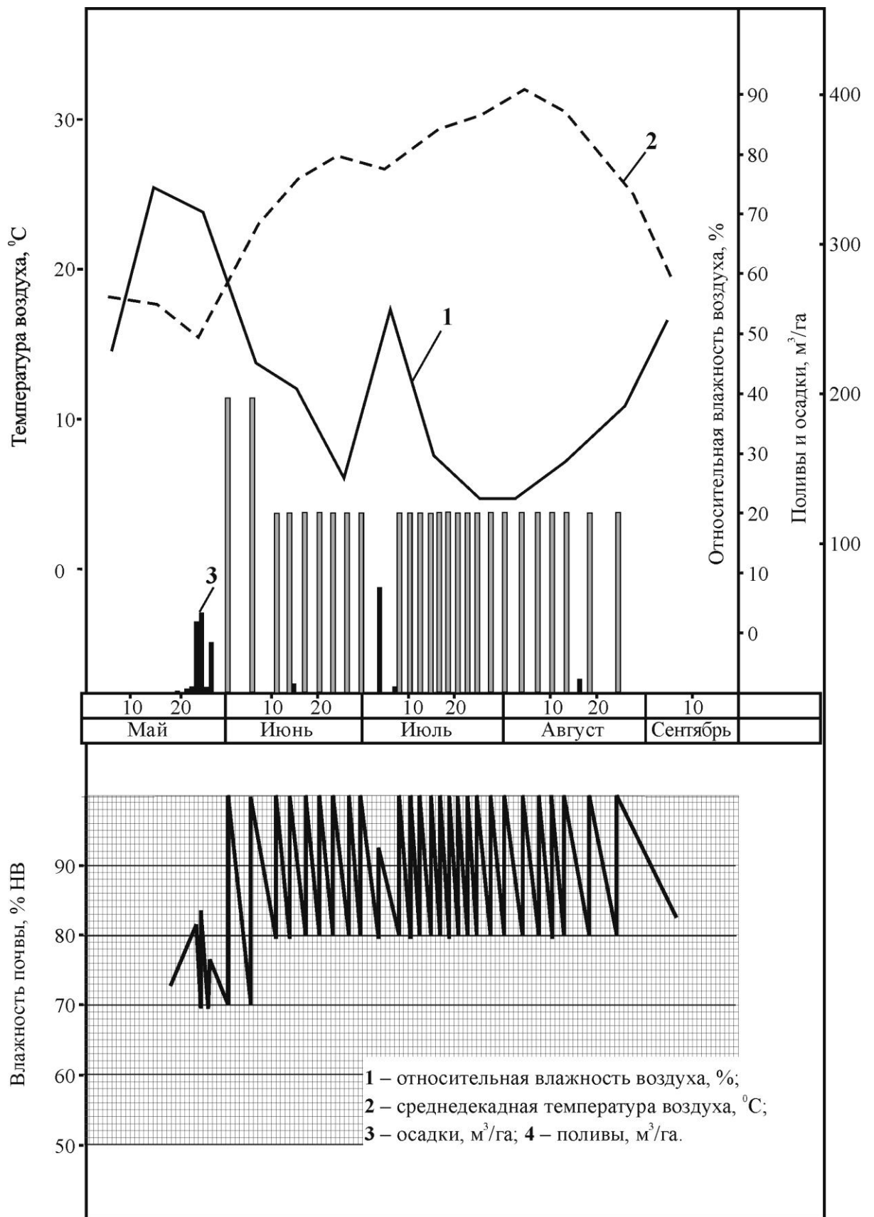
Рисунок 5.8 - Динамика изменения влагосодержания увлажняемой зоны почвогрунта в посевах сои ВНИИОЗ 86 для варианта поддержания предполивной влажности почвы 70-80-80 НВ (2010 г.)
