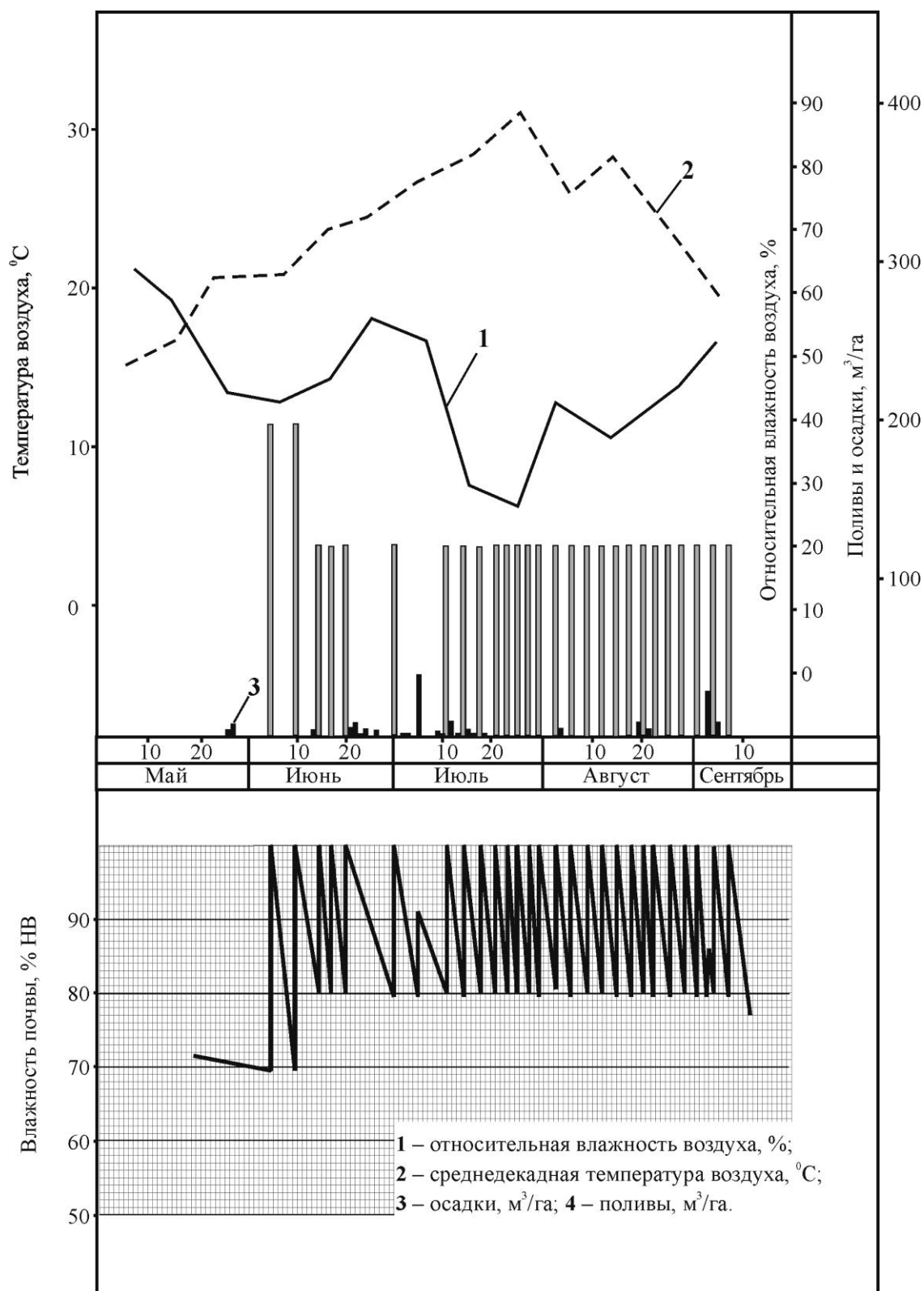
Рисунок 5.9 - Динамика изменения влагосодержания увлажняемой зоны почвогрунта в посевах сои ВНИИОЗ 31 для варианта поддержания предполивной влажности почвы 70-80-80 НВ (2011 г.)
